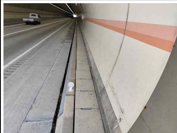
공동구 전경
